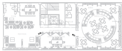
B1F樓監視平面配置圖
