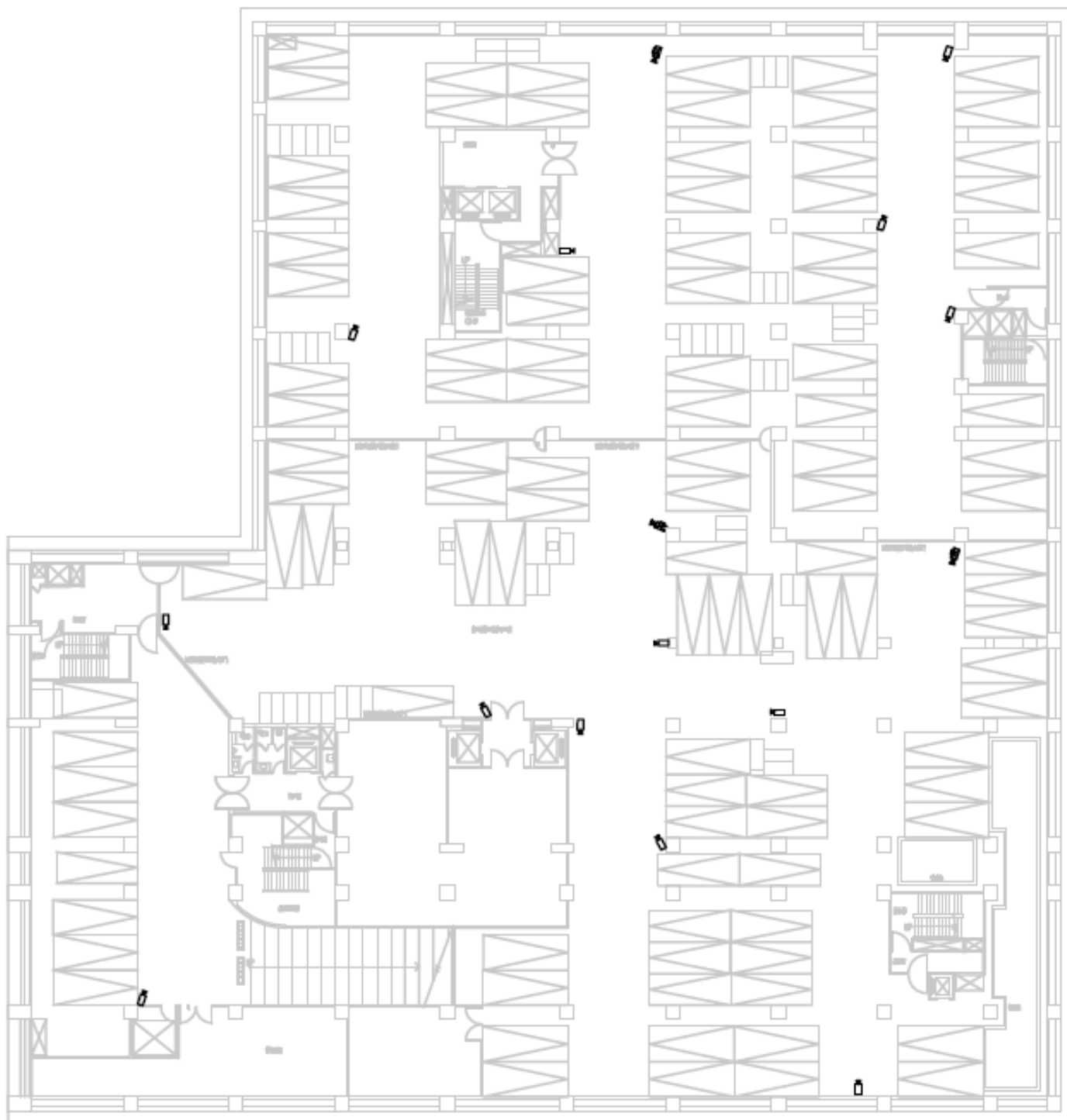
地下三層中央監控系統設備平面圖
