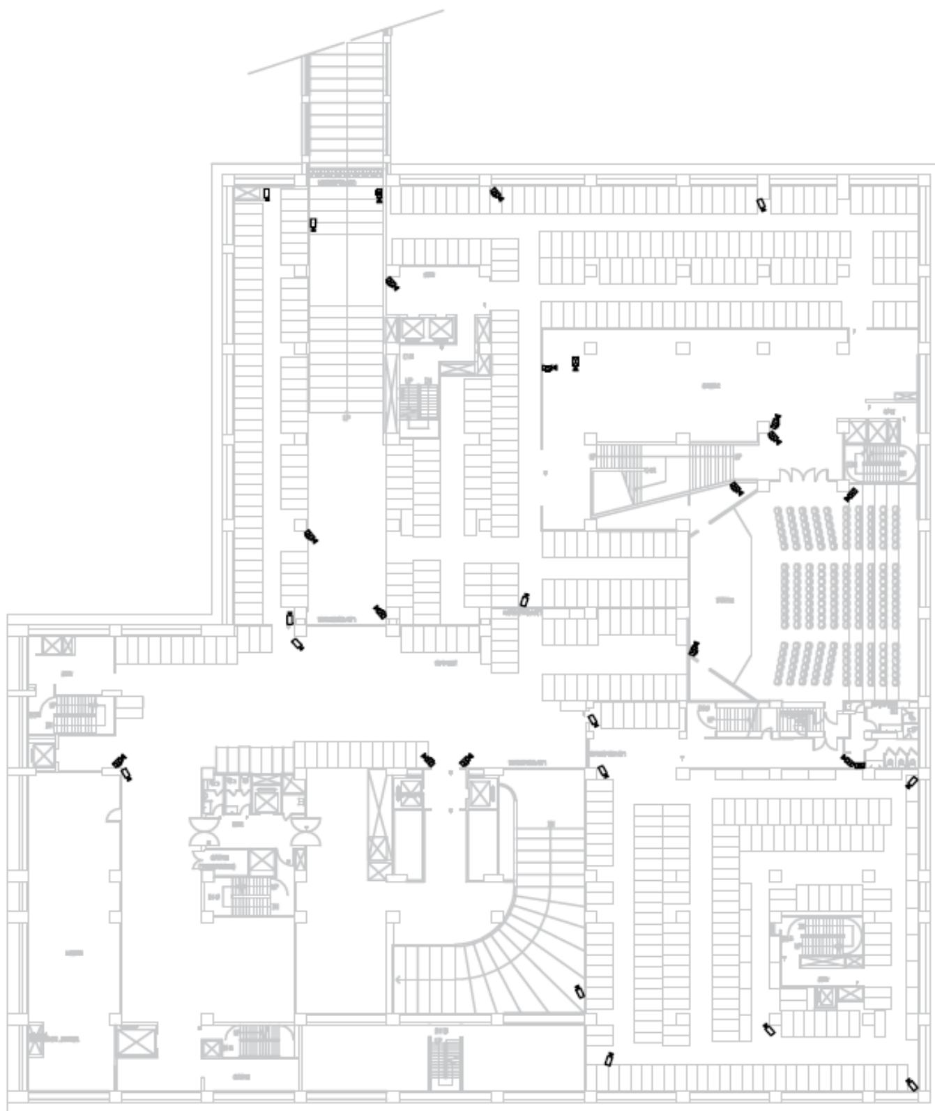
地下二層平面圖 S=1/200
